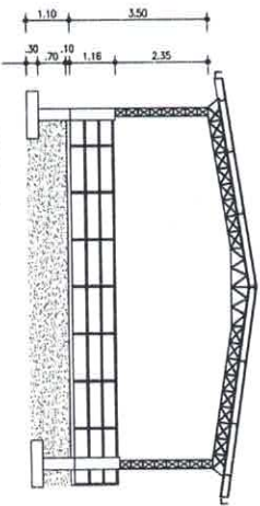
CORTE 01 ESC. 1:100
