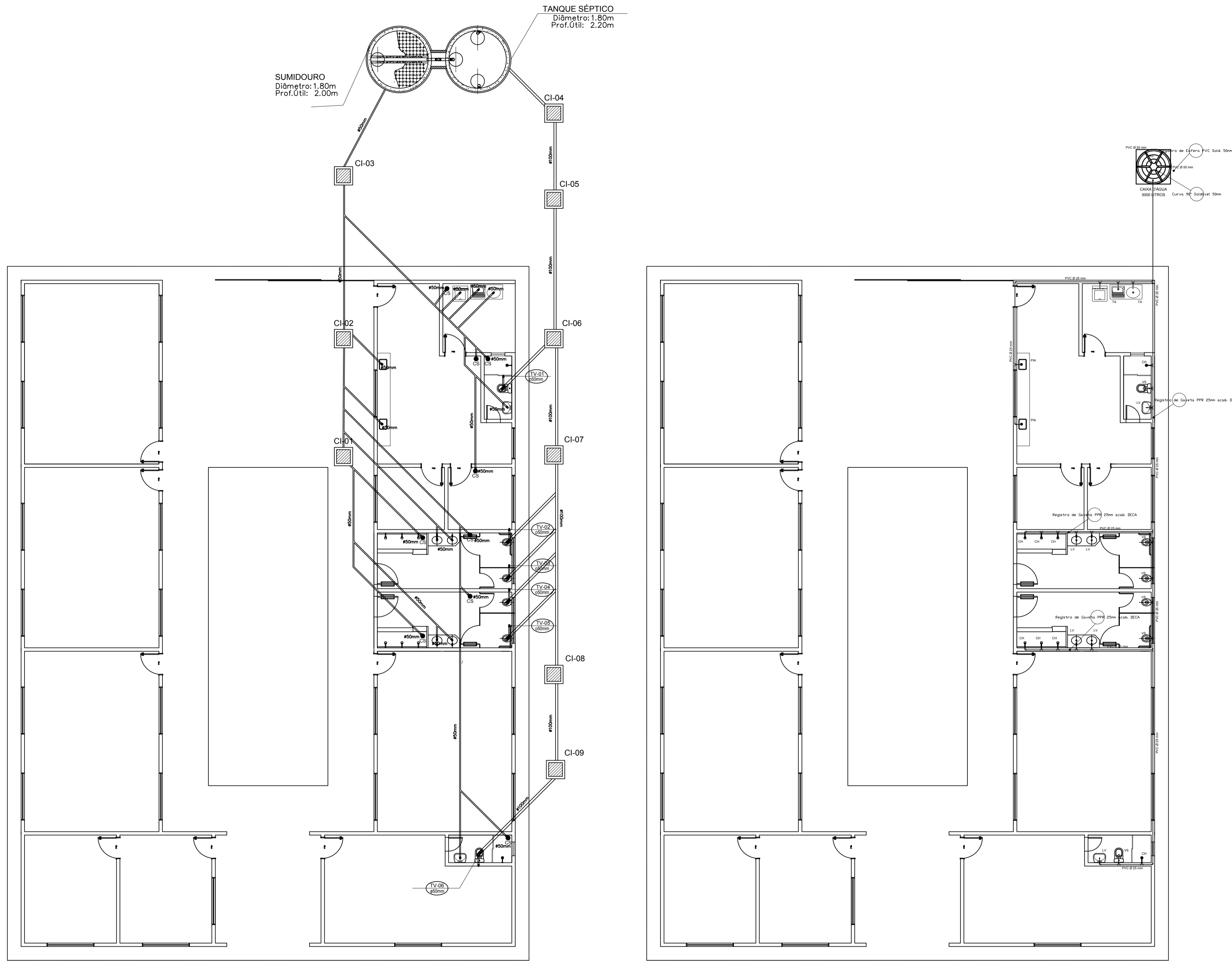
PLANTA HIDROSSANITÁRIA - CRECHE CASTELO DE SONHOS
