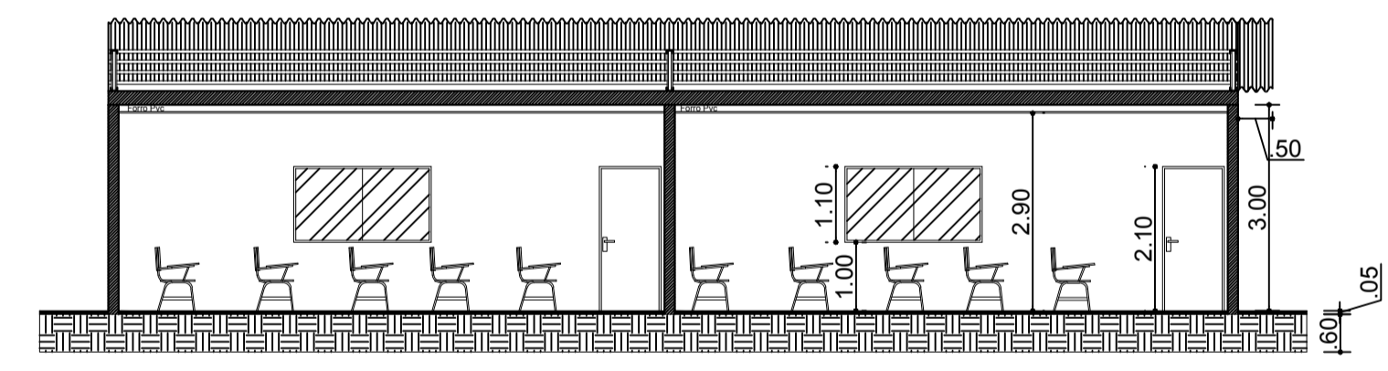
SEÇÃO TRANSVERSAL - SALAS ÁREA CONSTRUÍDA = 136,43 m 2 ESCALA: 1/75
