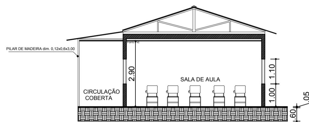
SEÇÃO TRANSVERSAL - SALAS ÁREA CONSTRUÍDA = 136,43 m 2 ESCALA: 1/75
