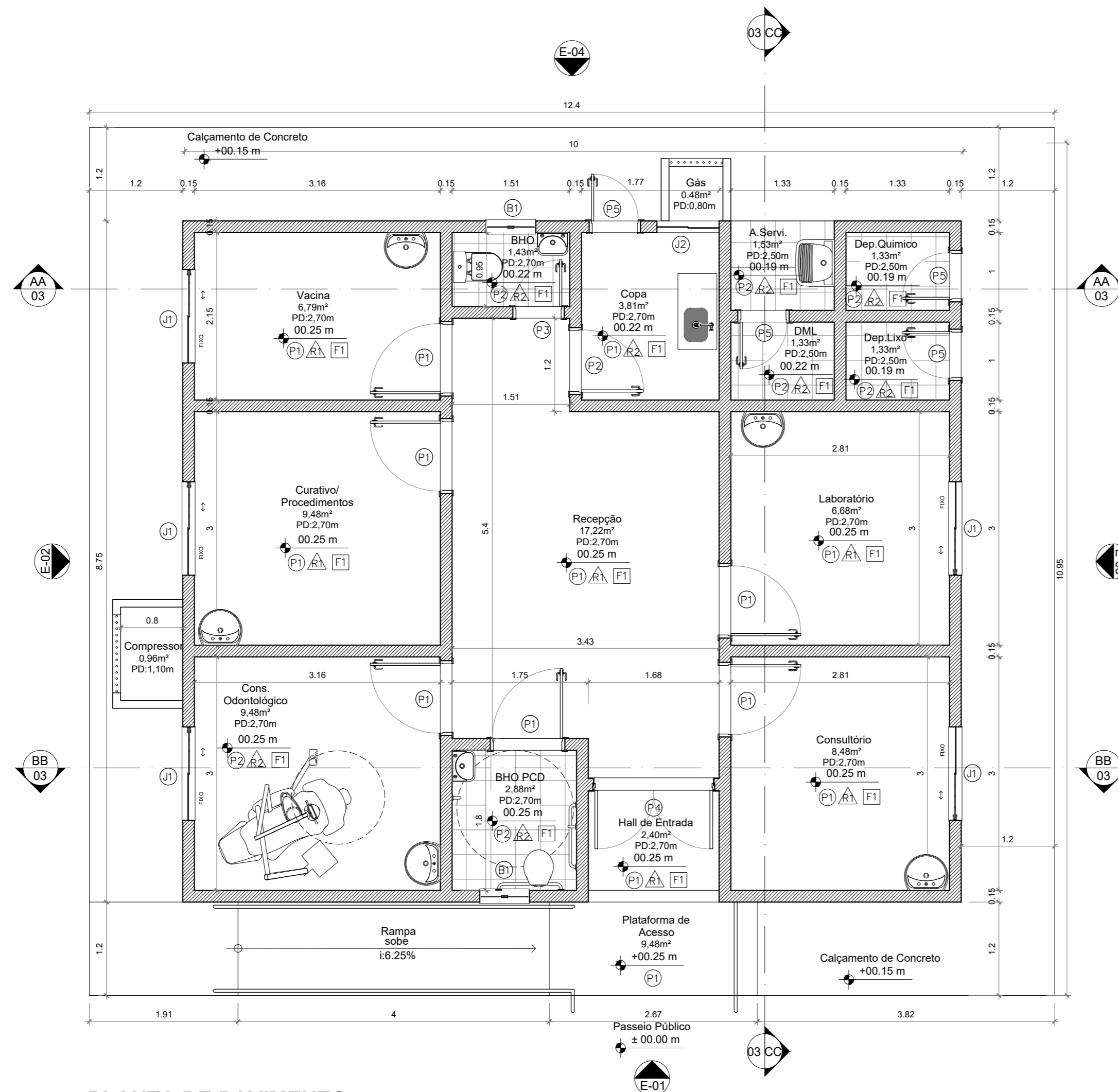
PLANTA DE PAVIMENTO UBS CANOPUS ESCALA - 1:50
