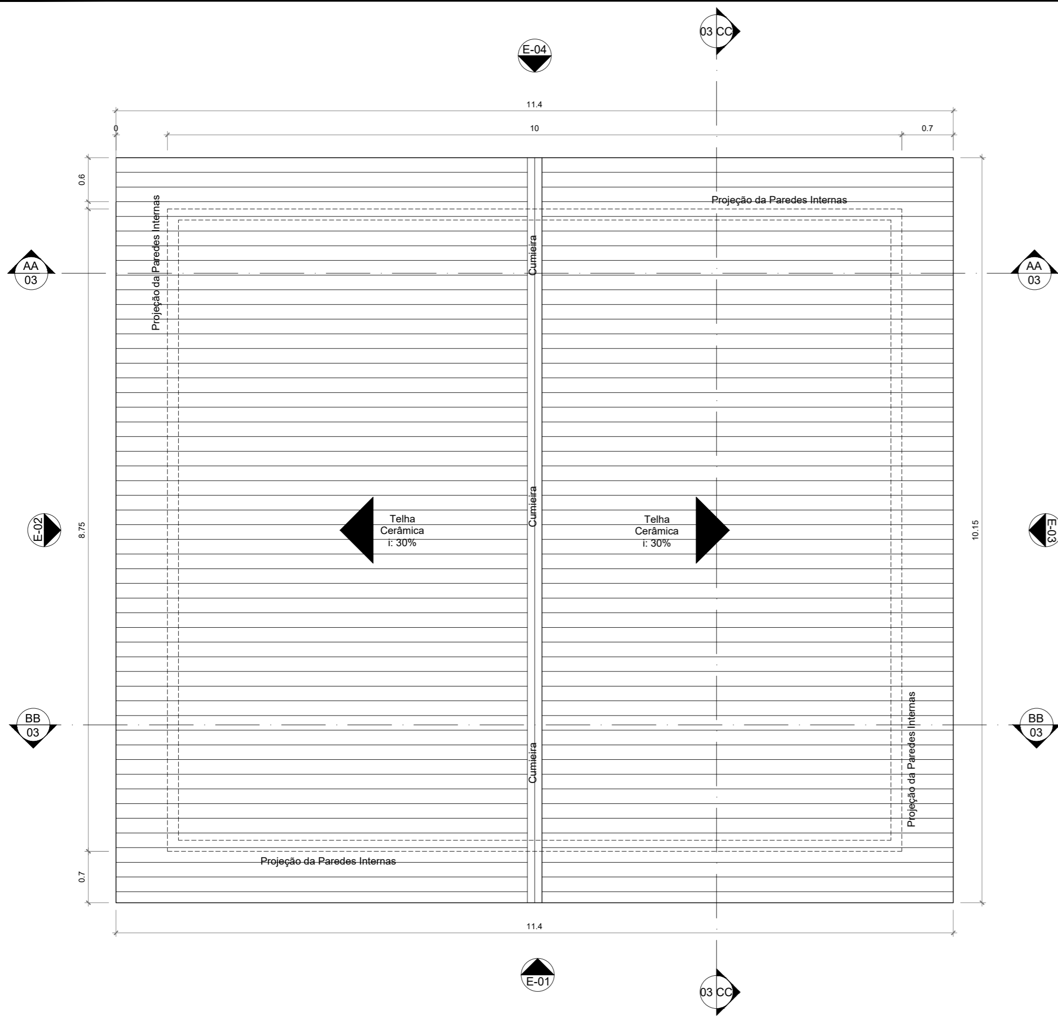
PLANTA DE COBERTURA UBS CANOPUS ESCALA - 1:50
