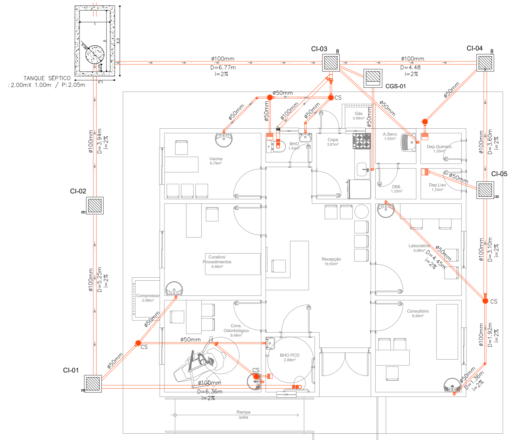
PROJETO DE ESGOTO UBS CANOPUS ESCALA - 1/75
