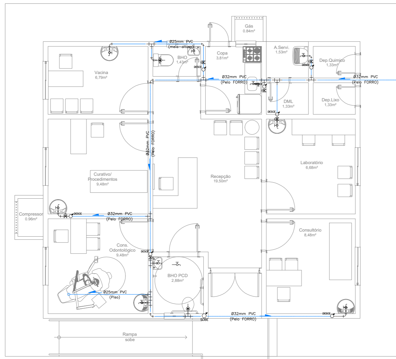
PROJETO HIDROSSANITÁRIO UBS CANOPUS ESCALA - 1/75
